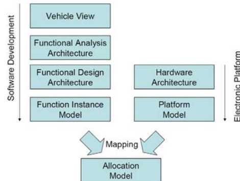
Abbildung 2: Abstraktionsebenen der EAST-ADL [Lö04]
