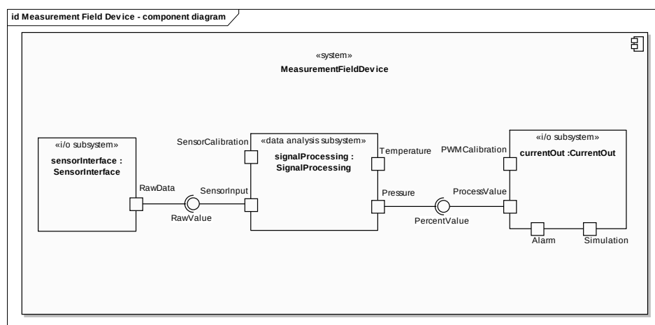
Abbildung 8: Komponentendiagramm für ein (sehr) einfaches Gesamtsystem
