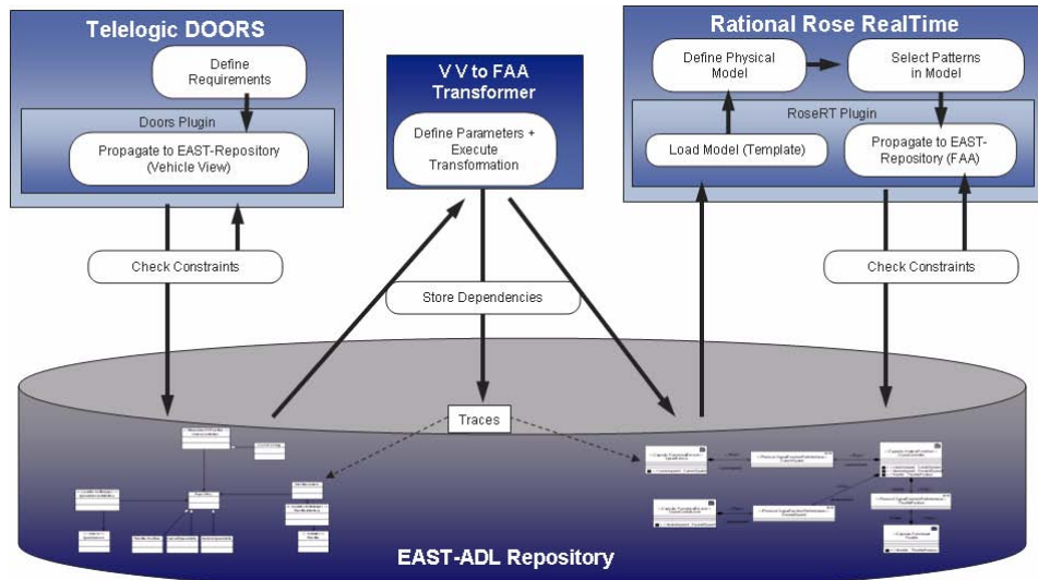
Abbildung 3: Entwicklungsprozess mit der Modell-Infrastruktur
