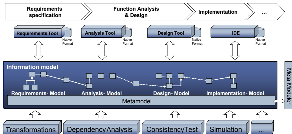
Abbildung 1: Das Architekturinformationsmodell
