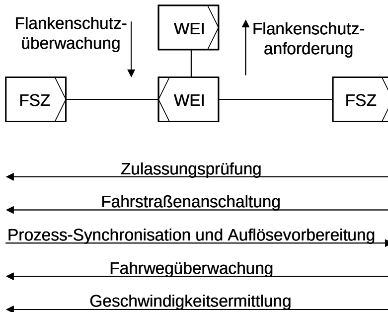
Abbildung 4: Komplexität der Kommunikation für einfache Steuerungsaufgabe
