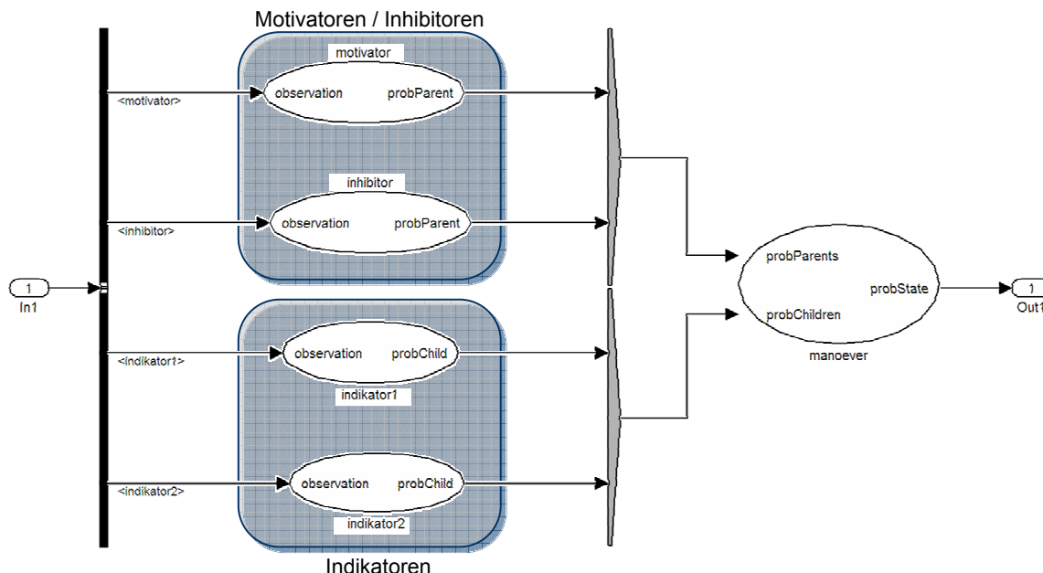
Bild 3: Aufbau eines Bayes'schen Netz mit Simulink
