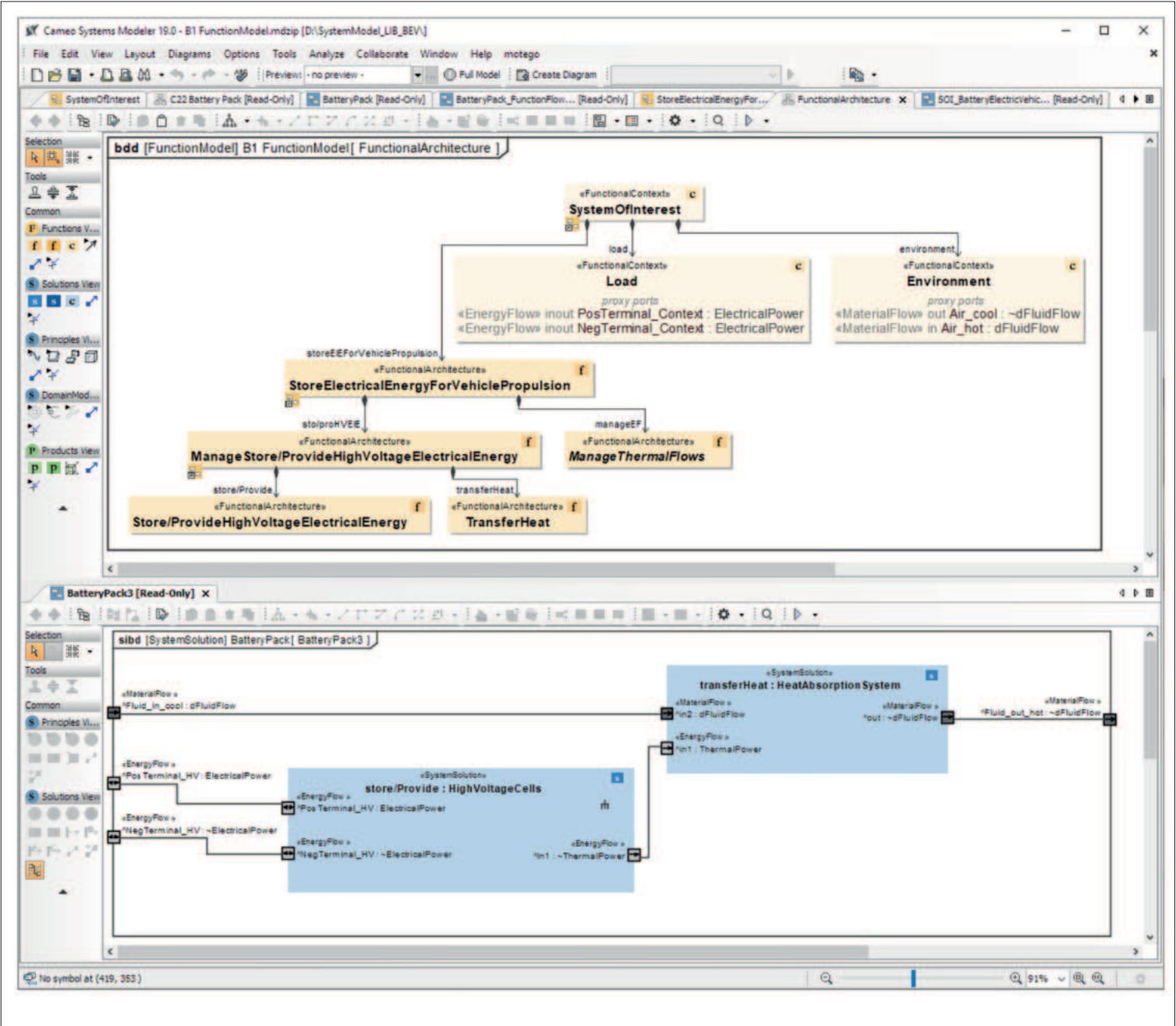
Bild 3: Mechatronisches System modelliert im motego-Sprachprofil
