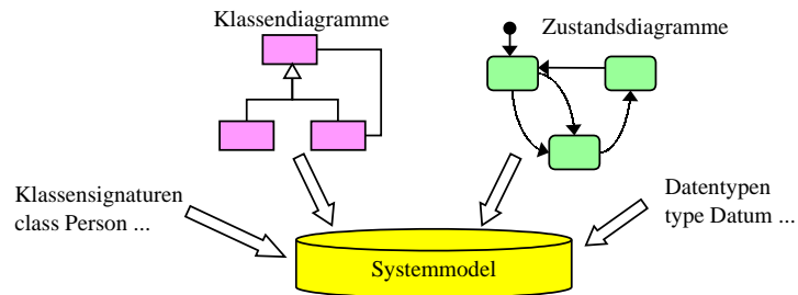
Abbildung 1: Formalisierte Dokumentarten
