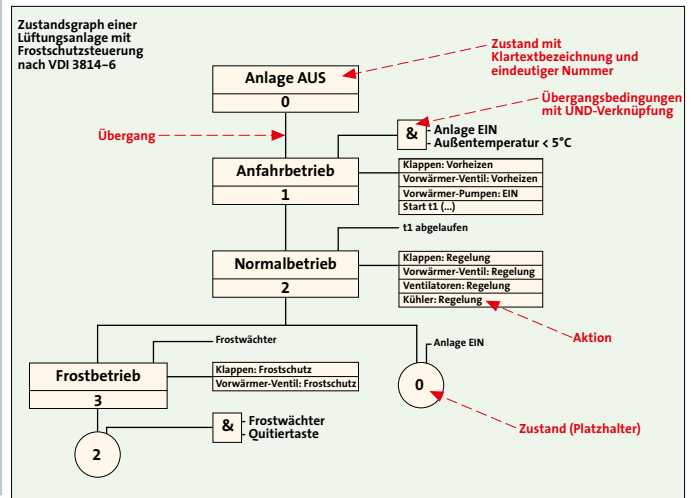
Bild 6: Beispiel für eine Zustandsgraphen für eine Lüftungsanlage nach VDI 3814 Beiblatt 6 [18]
